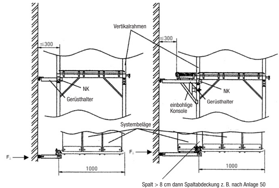
Bild 15 kurze Gerüsthalter
