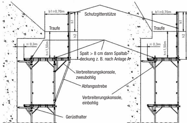
Bild 24 Dachfanggerüst (mit und ohne Verbreiterungskonsole)
