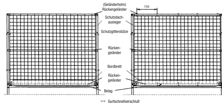
Bild 23 Schutzwand mit zugelassenen Schutznetzen
