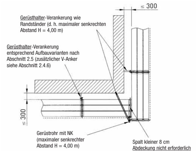
Bild 8b Eckausbildung ohne Spaltabdeckung
